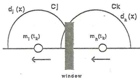
図6-3 1次元空間におけるLVQ2の動作原理。矢印は、参照用ベクトル m_j(t_k) と m_h(t_k) とが学習によって動かされる方向を示している。
