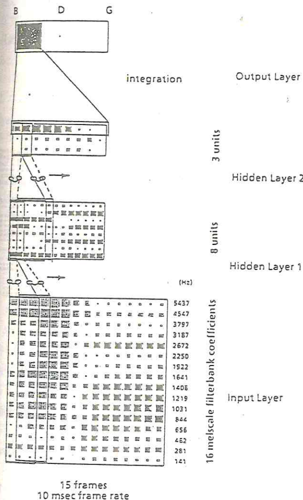
図 3-1 Time Delay Neural Network の構成
