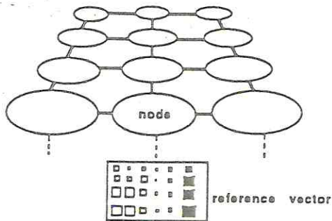
図6-1 2次元格子上的節点とこれに対応する参照用ベクトルの模式図。
