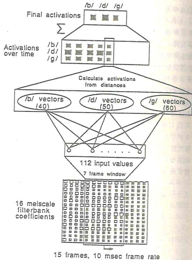
図6-5 Kohonen のネットワークを用いたシフトインバリエントな音韻認識システムの構成図。中間層の( )内の数字は、各音韻クラスごとの参照用ベクトルの数を示している。
