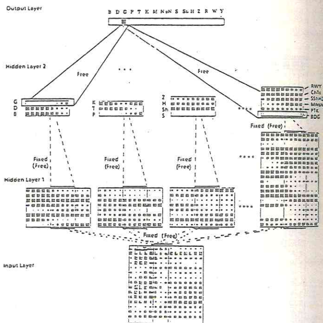
図 3-3 スケールアップされた全子音認識 TDNN の構成
