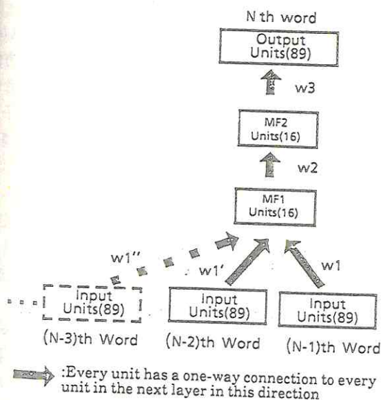
図 5-2 単語予測モデルの構成例
