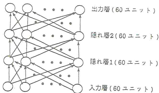
図4-1 雑音抑圧四層パーセプトロン
