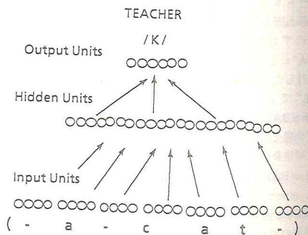
図5-1 NETtalk の構成
