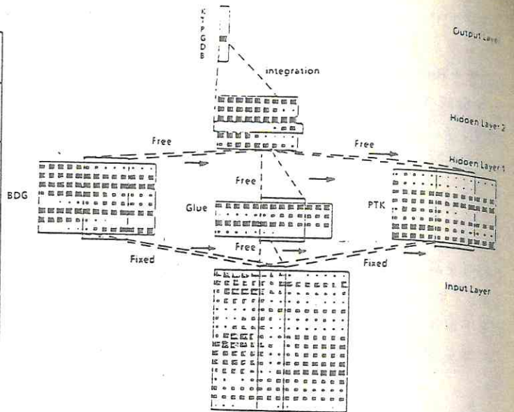
図 3-2 Connectionist Glue を持った Time Delay Neural Network の構成
