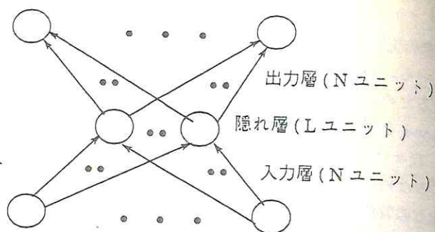
図4-2 情報圧縮三層パーセプトロン ( L < N )
