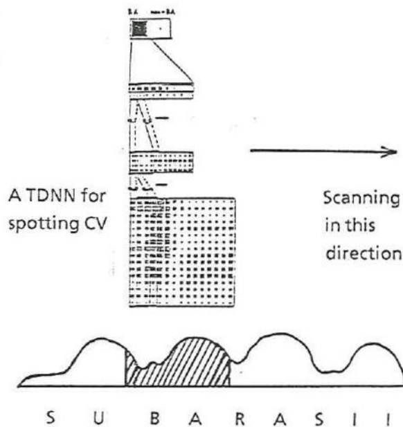
図 2. 単音節のスポッティング実験
