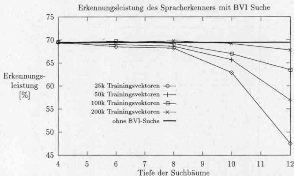
Abbildung 35: Auswirkungen der Anzahl der verwendeten Trainingsvektoren und der Tiefe der Suchbäume auf die Erkennungsleistung des Spracherkenners
