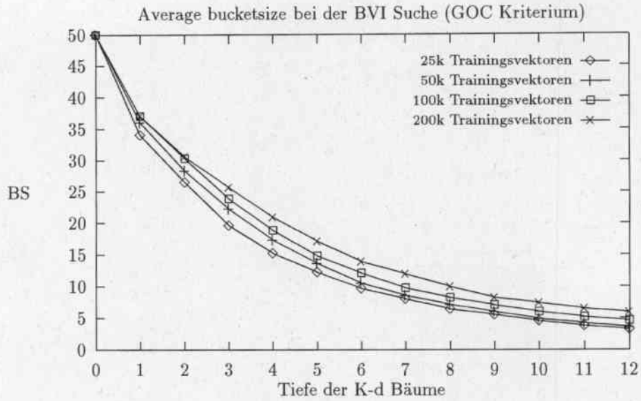
Abbildung 20: Average bucketsize beim GOC Kriterium
