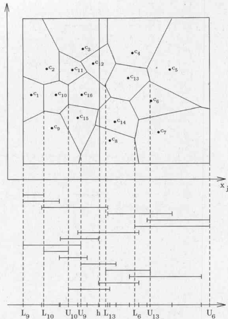
Abbildung 9: Voronoi-Projektionen zur Bestimmung von n_L und n_R
