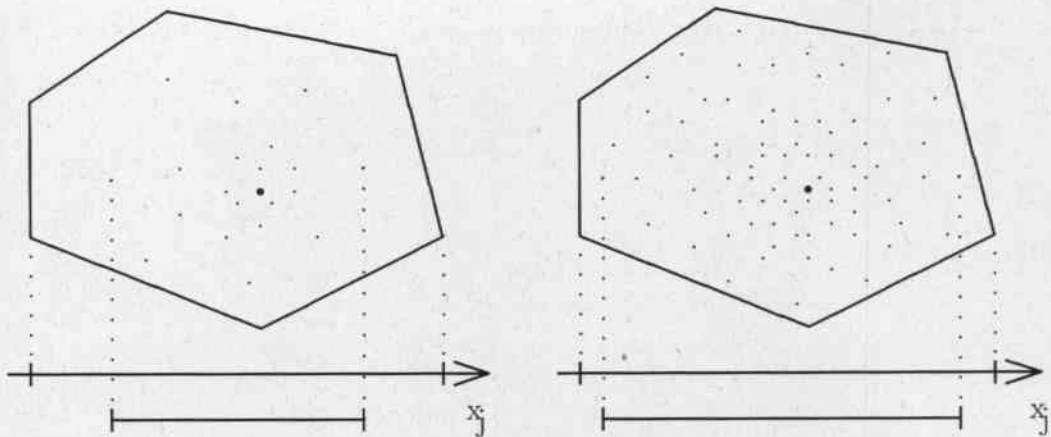
Abbildung 14: Approximation der Projektion des Voronoi-Gebietes eines Codebuchvektors mit wenigen (links) und vielen (rechts) Trainingsvektoren
