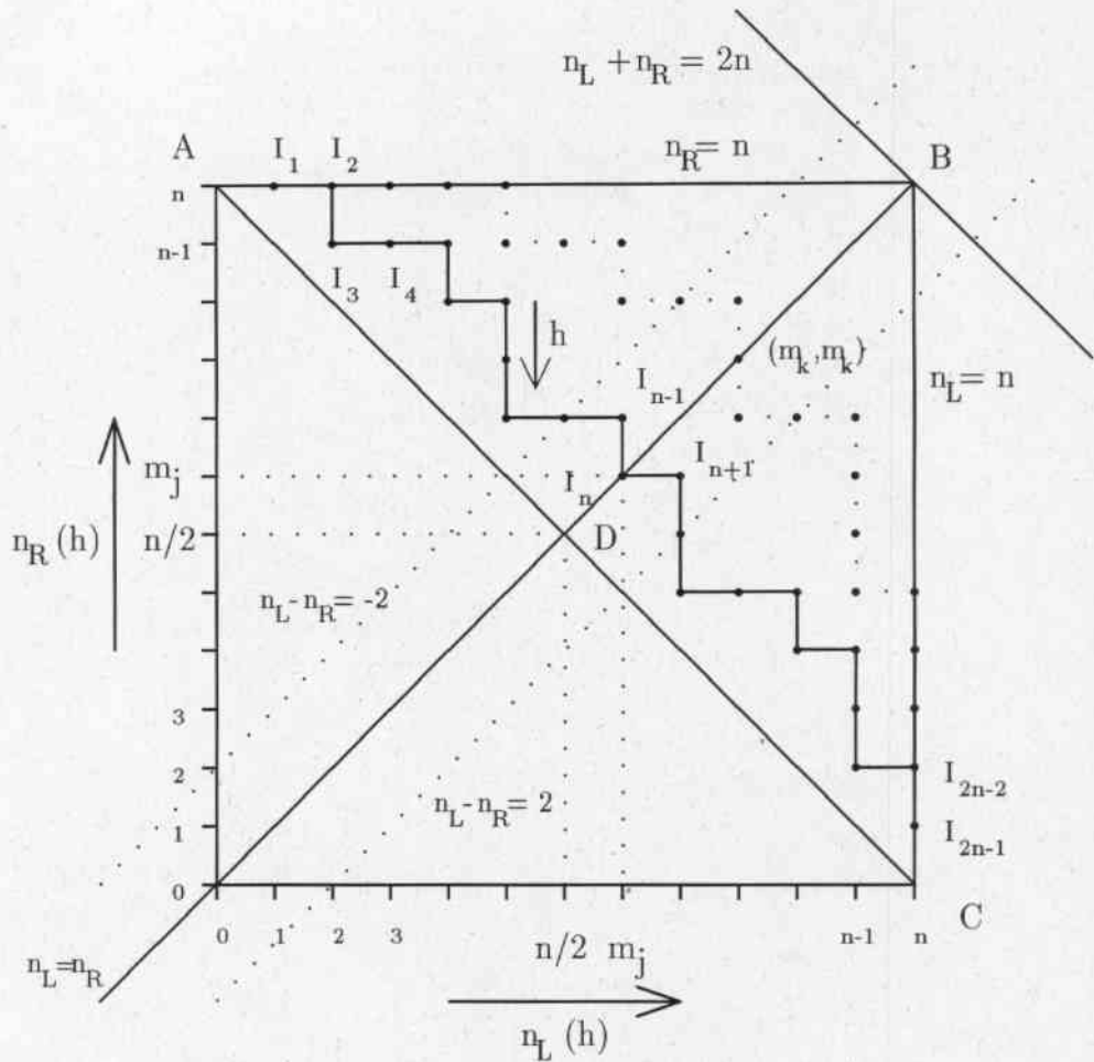
Abbildung 11: Geometrische Interpretation des GOC Optimierungskriteriums dargestellt in der n_L-n_R -Ebene
