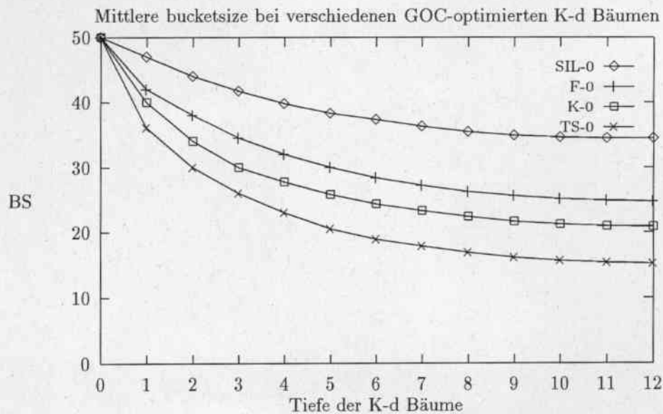
Abbildung 30: Mittlere bucketsize bei der approximativen Optimierung
