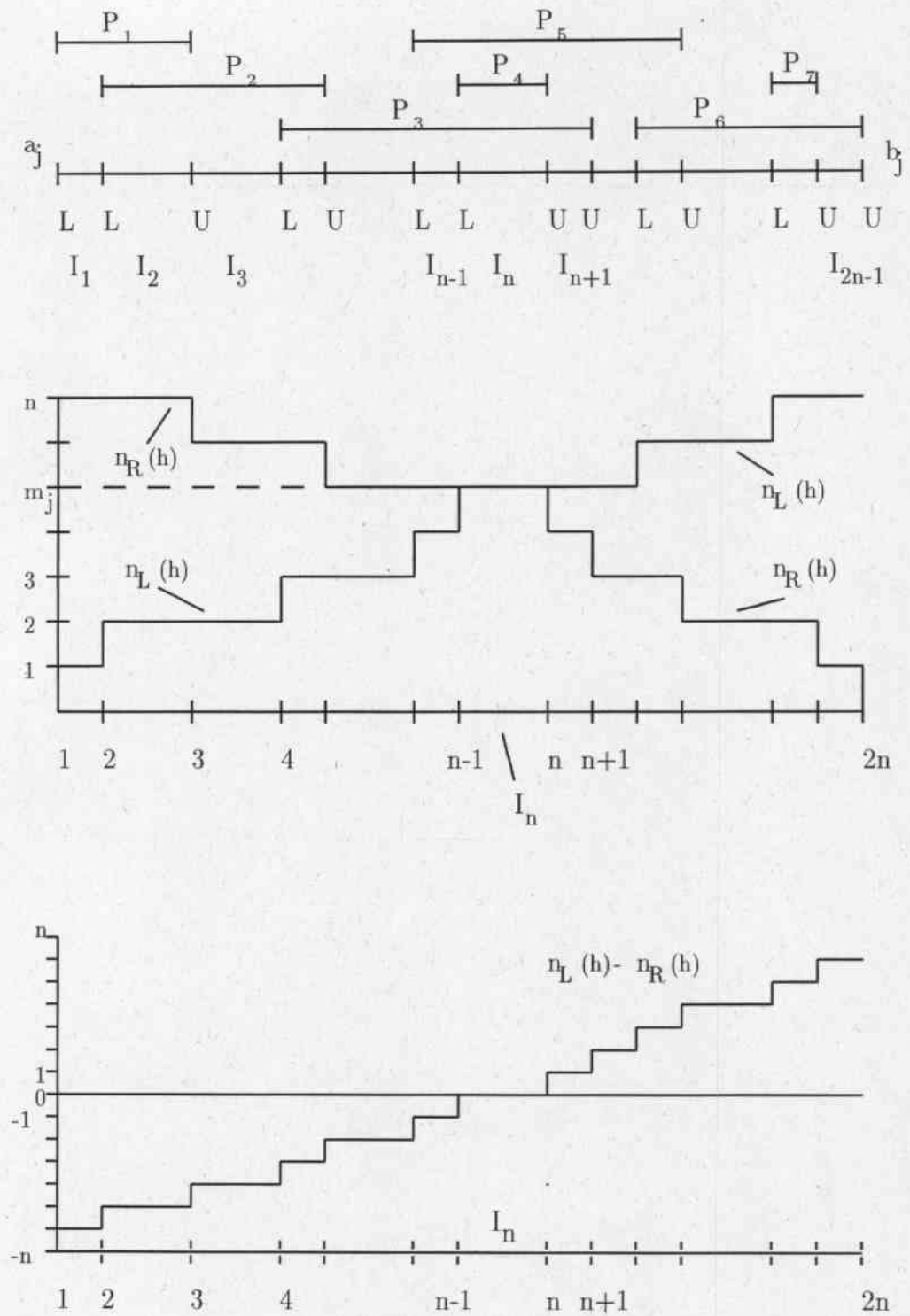
Abbildung 10: Typischer Verlauf der Funktionen n_L, n_R und (n_L - n_R) zu gegebenen Voronoi-Projektionen, abhängig von der Position h der Trennhyperebene
