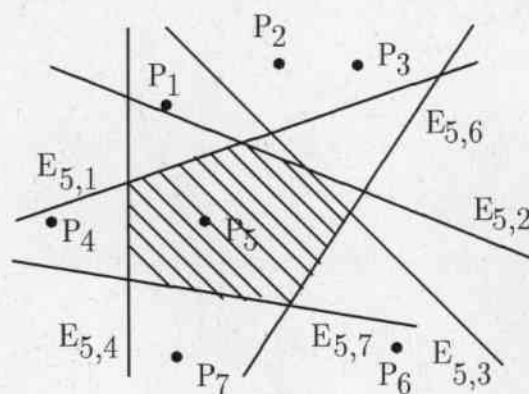
Abbildung 2: Voronoi-Gebiet eines Punktes im \mathcal{R}^2
