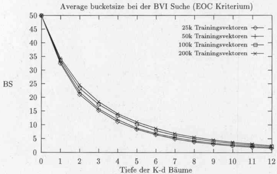
Abbildung 21: Average bucketsize beim EOC Kriterium
