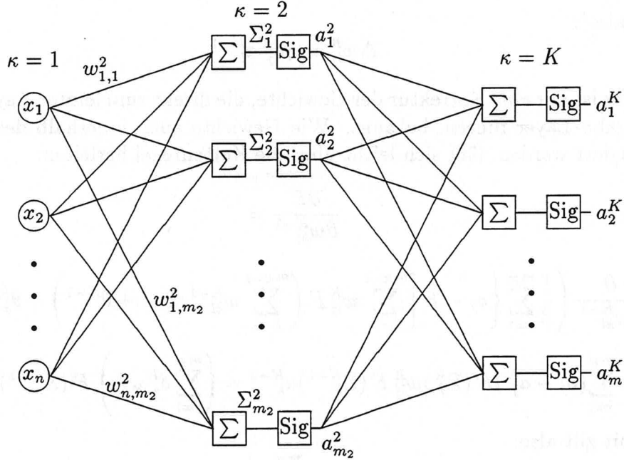
Abbildung A.1: Bezeichnungen des neuronalen Netzes
