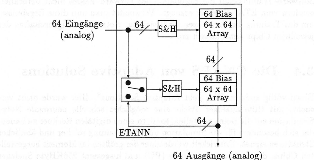
Abbildung 3.3: Blockschaltbild des ETANN-Chips von Intel.
