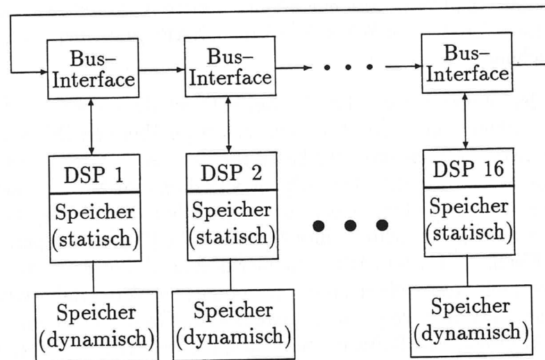
Abbildung 3.5: Blockschaltbild der RAP (16 Knoten)
