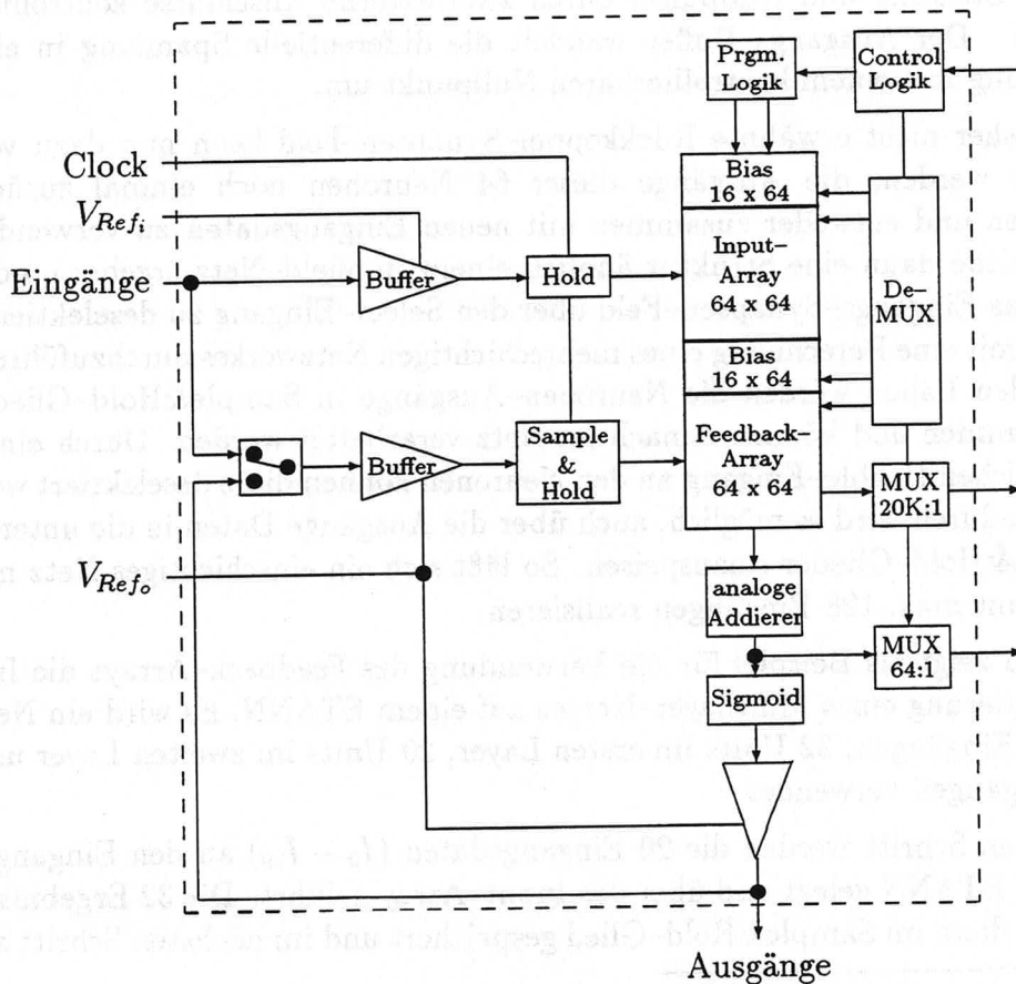
Abbildung 5.2: Blockschaltbild des ETANN
