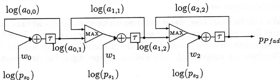
Abbildung 7.5: Das Netz zur Berechnung des Viterbi-Algorithmus
