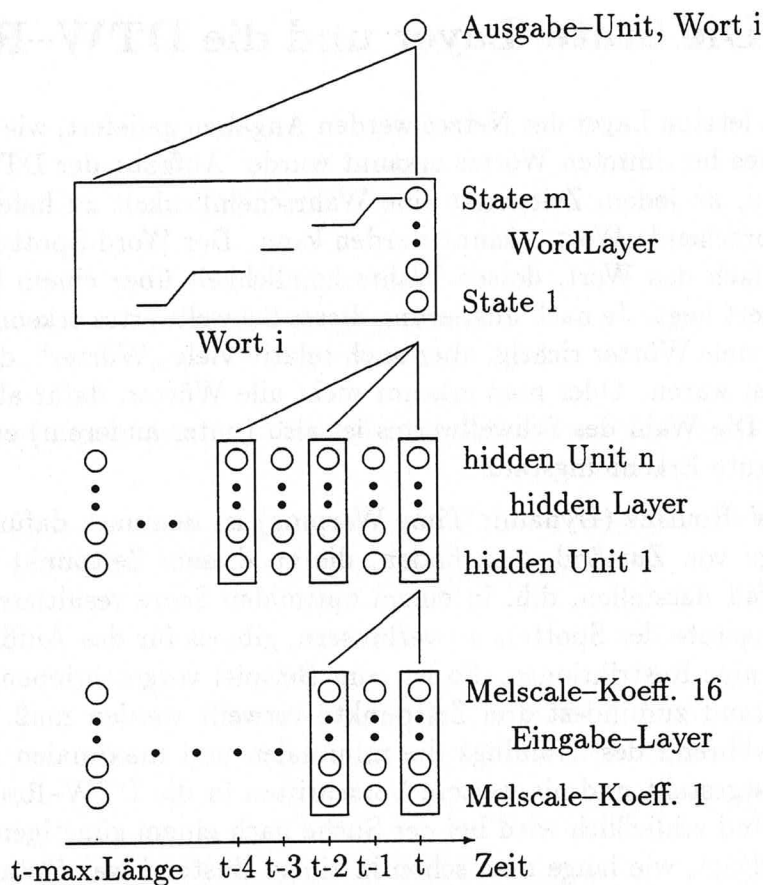
Abbildung 6.1: Die Struktur des WordSpotters
